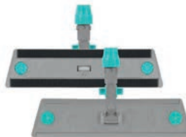
Telaio con sistema a strappo e dischi fermapanno ovali con block system
